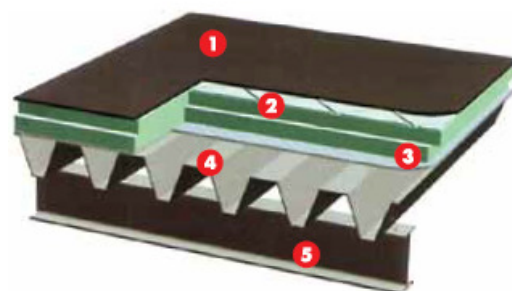
Dach płaski - blacha trapezowa
