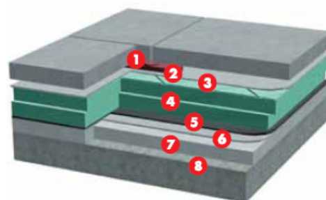
Parking - dach odwrócony - powierzchnia z elementów gotowych
