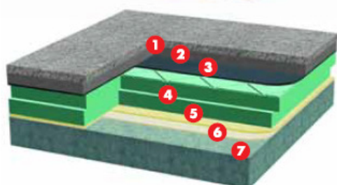
Posadzka przemysłowa na gruncie
